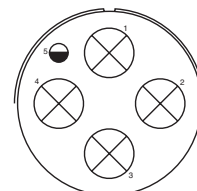
40-75 4-#0; 1-#12 ● ⊙ E
