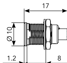
Front Mount (ER)
